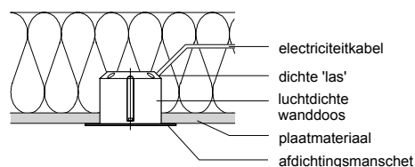
89. Een luchtdichte uitvoering van een wandcontactdoos.
