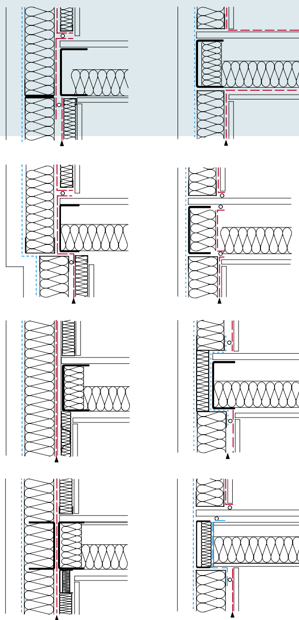
93. Verschillende aansluitingen van vloeren op buitenwand voor de balloon- en platformmethode met lucht- en winddichte uitvoeringen. De rode folie is dampremmend, de blauwe folie is dampdoorlatend.
