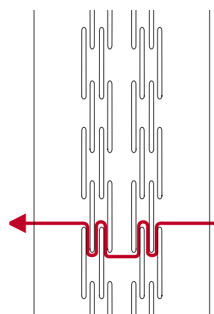
81, 82. Een 'thermoprofiel'. De sleuven in het lijf verlengen de 'weg' van de warmtestroom en voorkomen koudebruggen.
