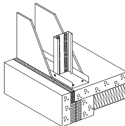
85. Funderingsdetail met thermoprofielen.
