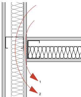
60. Geluidoverdracht via het flankerende bouwdeel:
