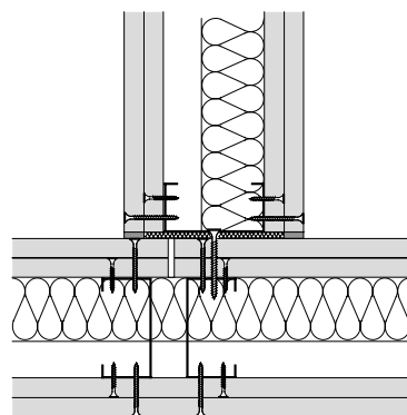
62. Akoestisch 'goed' gedetailleerde wandaansluiting met gesloten voeg en een scheiding in de doorgaande bekleding.
