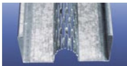
52. Akoestisch metal-studprofiel uit strekmetaal.
