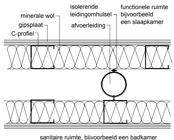
73. Verticale leiding in een dubbele wandconstructie.
