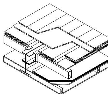
58. Vloerbouw met een driedubbele ontkoppeling van de bekleding.
