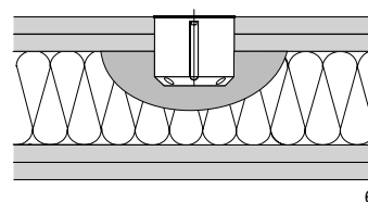
104. 'Protocol' voor het inbouwen van wandcontactdozen en wanden met een brandwerende functie.
