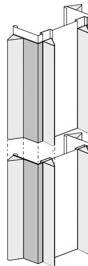
63. Metal-studprofiel met droge, rubberen geluidprofielen.
