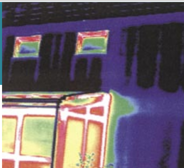
79. Thermovisuele weergave van een staalframebouw woning.
