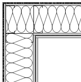
vergroete koudebrug door gekoppelde profielen
