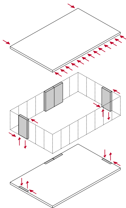
12. Stabiliteit uit schijfvormige wand- en vloerelementen.
