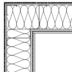
verbeterde koudebrug door gescheiden constructie
