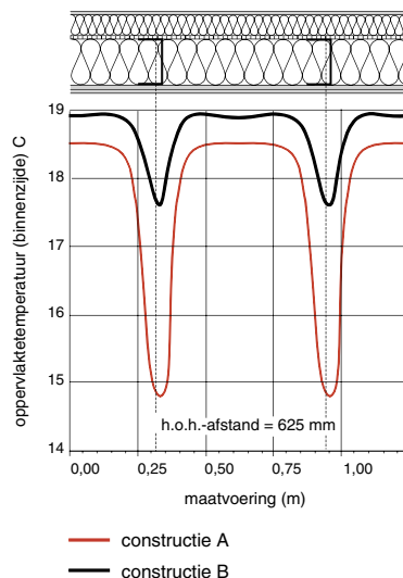
78. Koudebruggen: de invloed van de stijlen op de oppervlakte temperatuur aan de binnenzijde.
