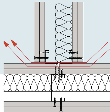
61. Akoestische 'lekken' en geluidbruggen bij een aansluiting van twee wanden.
