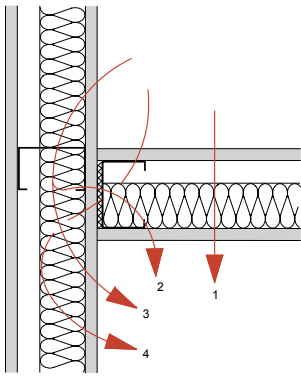
59a. Geluidoverdrachtswegen in staalframebouw en massieve bouw zijn vrijwel gelijk.
