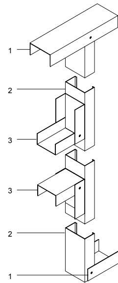
1 regels van U-profielen 2 stijlen van C-profielen 3 kalven van U-profielen
