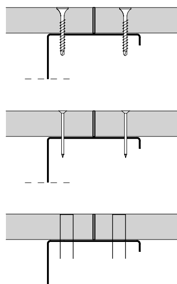
45. Verbindingsmogelijkheden van een beplating op staal framebouw.
