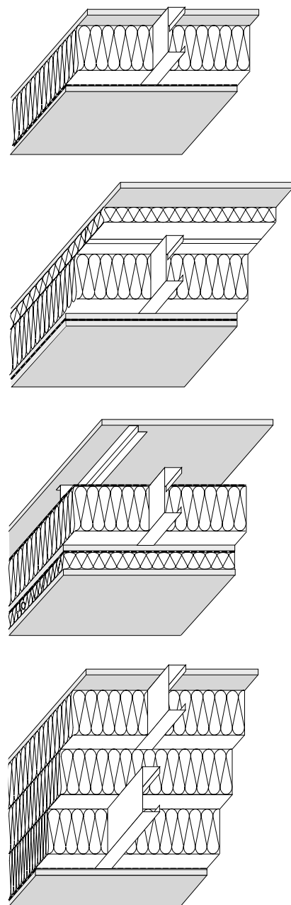
74. Verschillende opbouwen van staalframebouw wanden.
