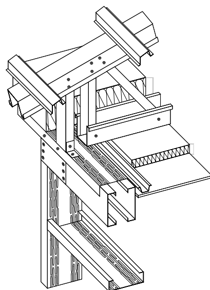
84. Dakdetail met thermoprofielen.
