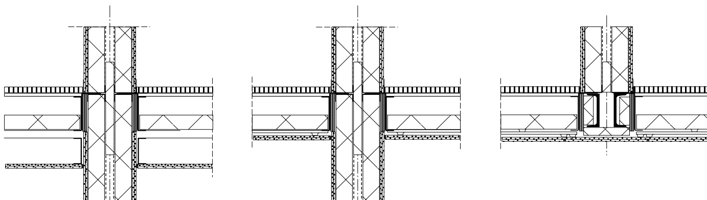
65. Detailoplossingen met L_{\infty} > +5 dB.
